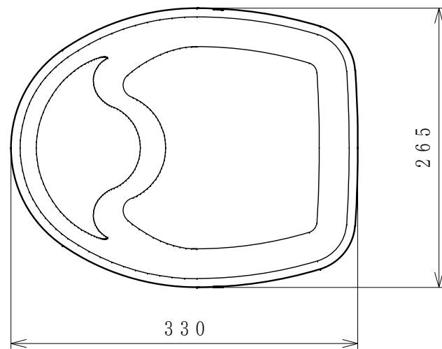
バケツ外形
