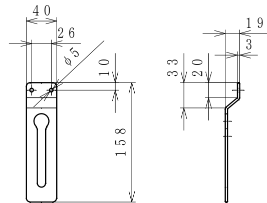
固定金具
